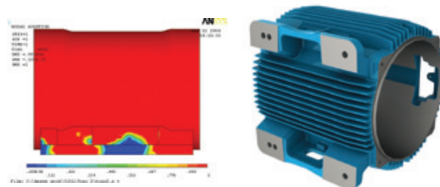
Figura 4 - Patas sólidas
